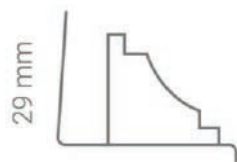
B4 Stropní ukončovací lišta
